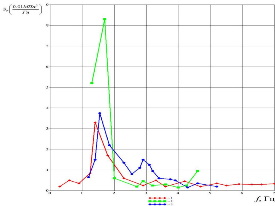
1 – эксперименттегі жазба бойынша; 2 – профильді тегістеу ұзындығымен l = 25 мм; 3 – тегістеу ұзындығы бойынша l = V/f_H 4. сур. Троллейбус рамасының ланжерон кимасындағы кернеудің спектрлік тығыздығы № 5, V=30 км/сағ сенсор) есептелген
